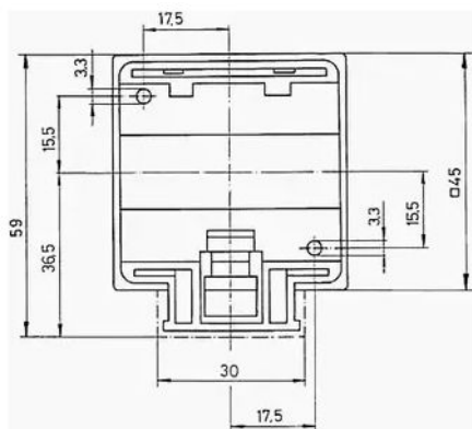
Masszeichnung-1
