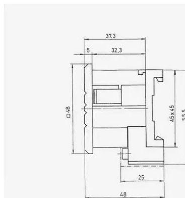
Masszeichnung-2
