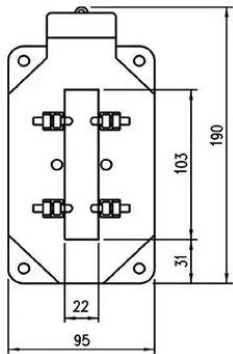
Masszeichnung-1
