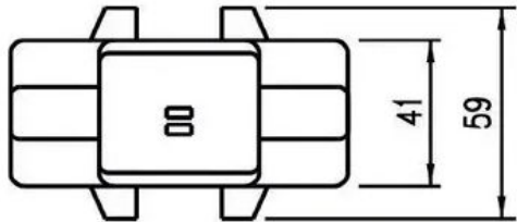
Masszeichnung-2
