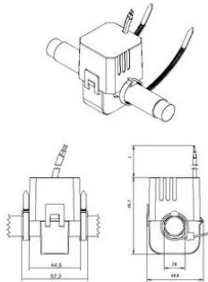
Masszeichnung-2
