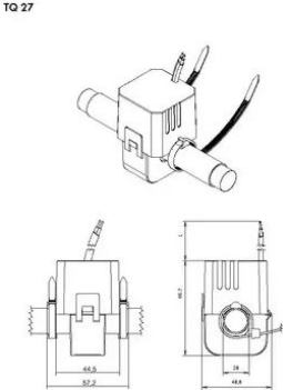
Masszeichnung-2
