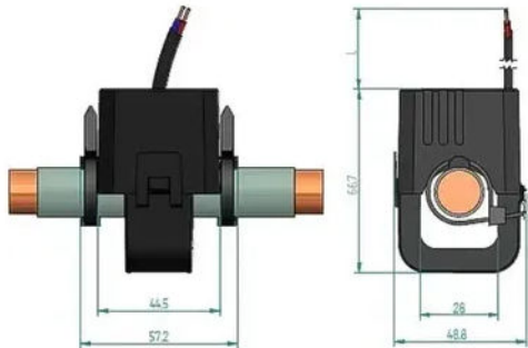
Masszeichnung-1
