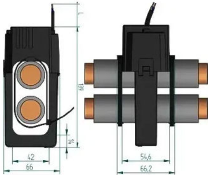
Masszeichnung-1
