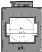
Plano de dimensiones 2
