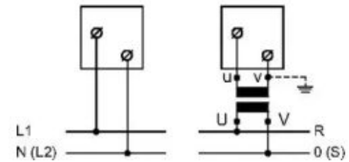
Esquema de conexión 1
