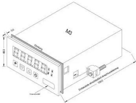
Plano de dimensiones 1
