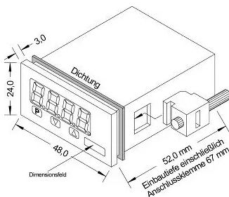
Maßzeichnung 1
