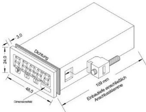
Maßzeichnung 1
