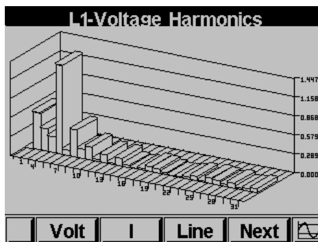
Abbildung 5.10 Oberwellen-Balkendiagramm
