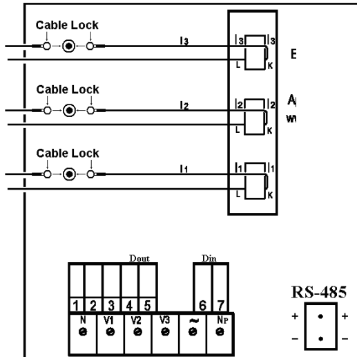
Abbildung 2.5 Rückseite
