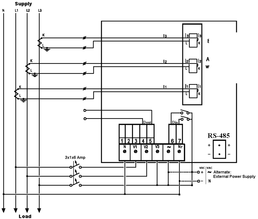
Abbildung 2.3 Verdrahtungsschema „Stern“-Schaltung
